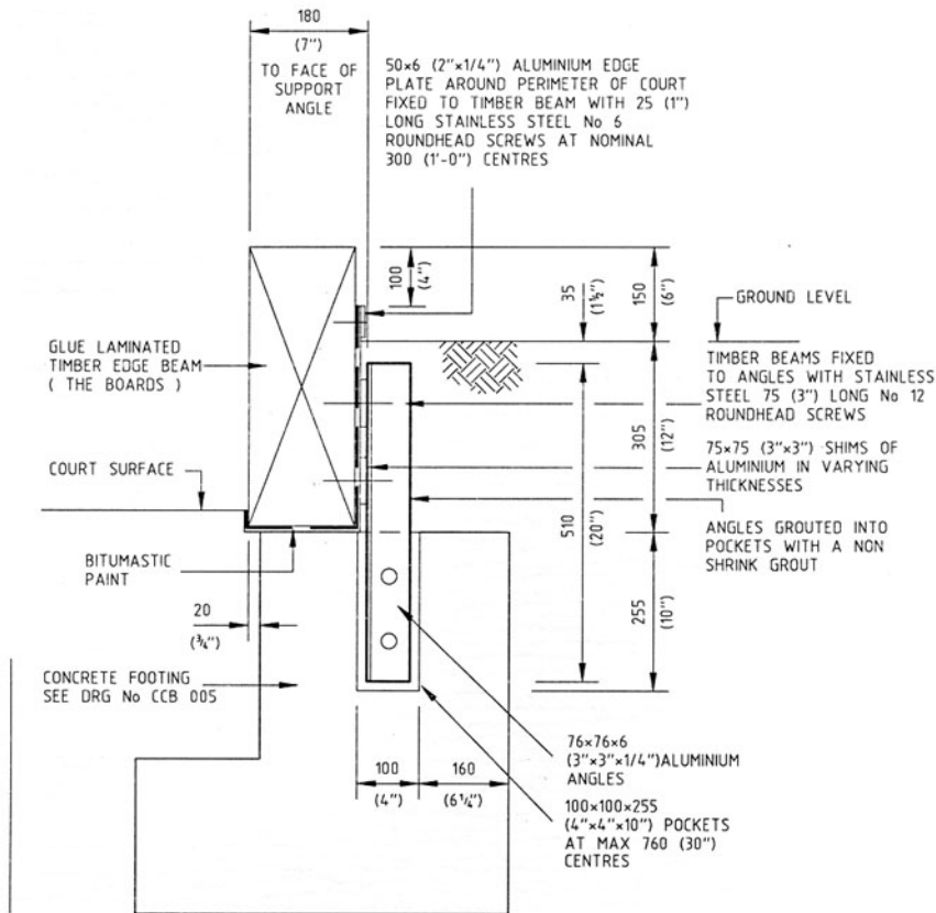
COURT EDGE DETAIL
