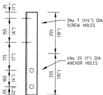
ANGLE FABRICATION
